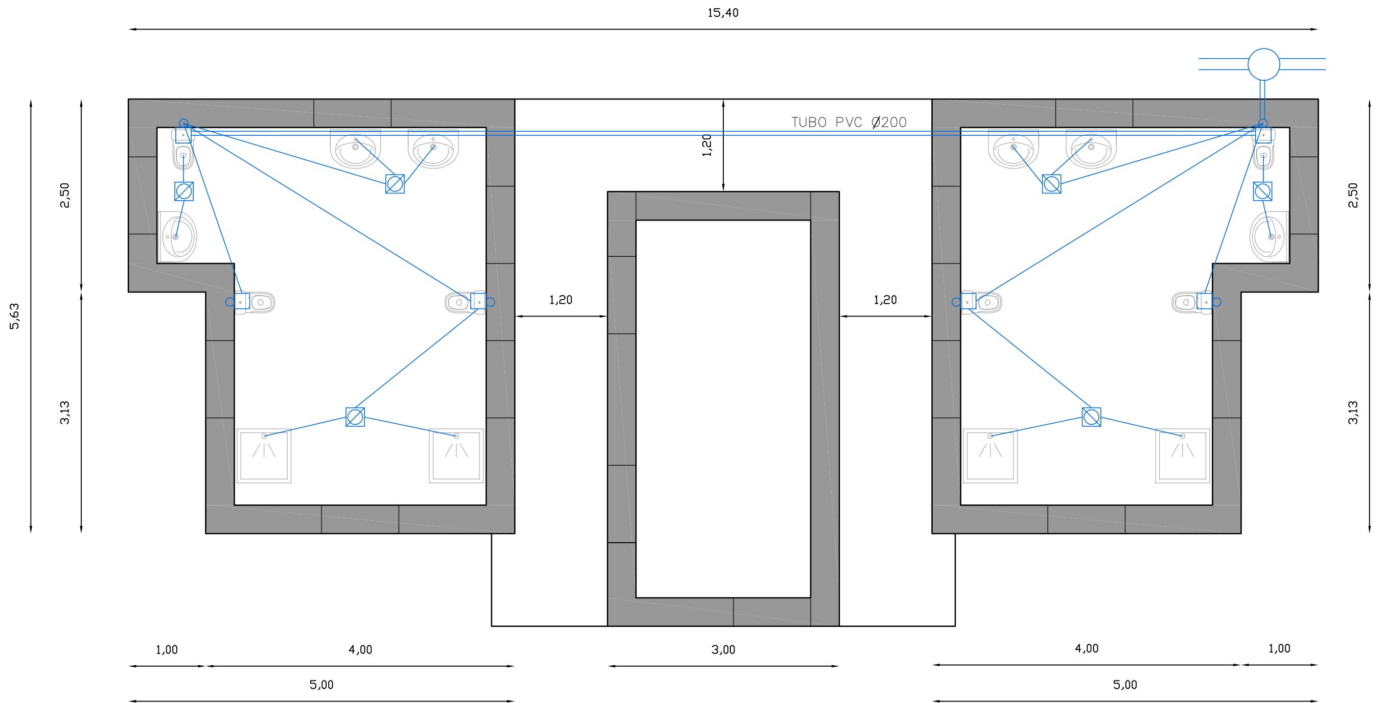
PLANTA DE CIMENTACION Y SANEAMIENTO
