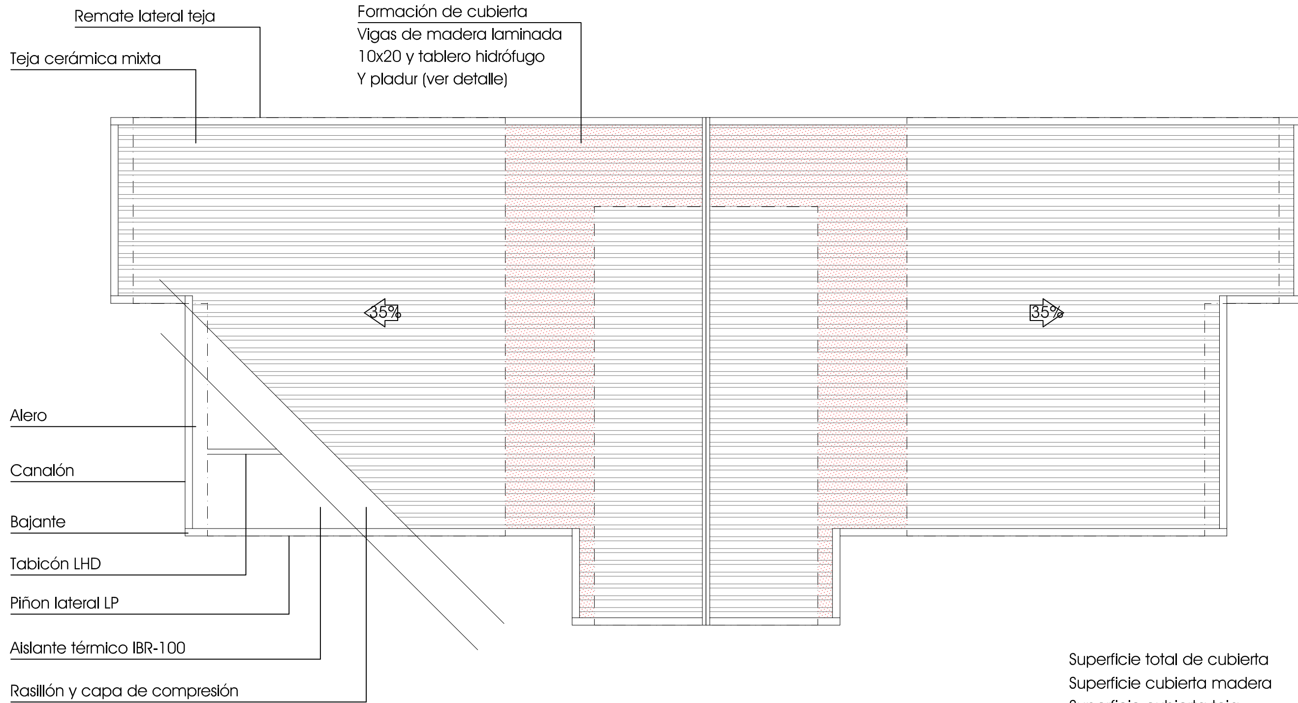
PLANTA DE CUBIERTA Y FORMACION DE CUBIERTA
